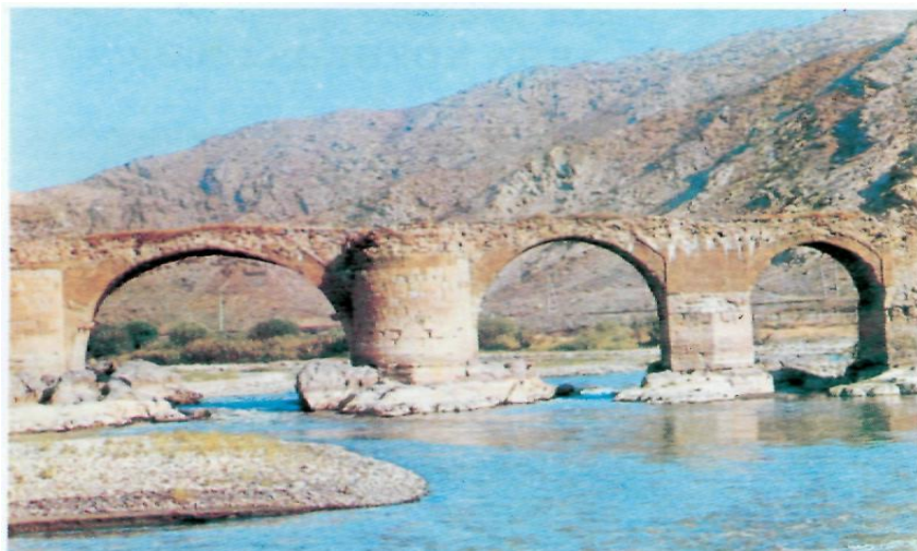
On bir aşırımlı Xudafərin körpüsü
